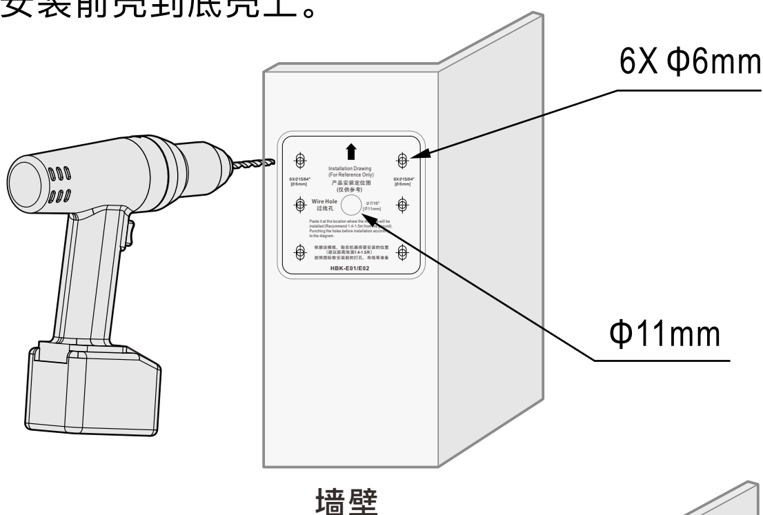
图2-安装膨胀管
